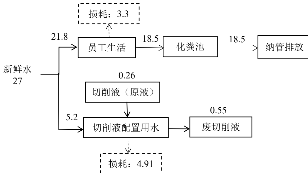
图 2-1 项目调试期间水平衡图
