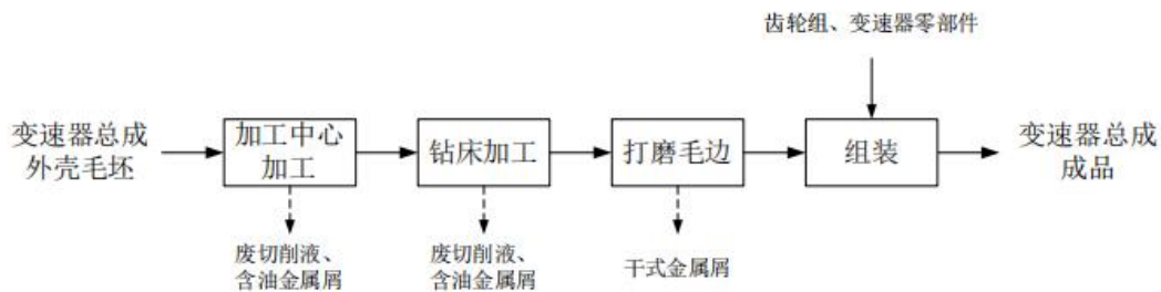
图 2-4 变速器总成生产工艺流程及产污图
