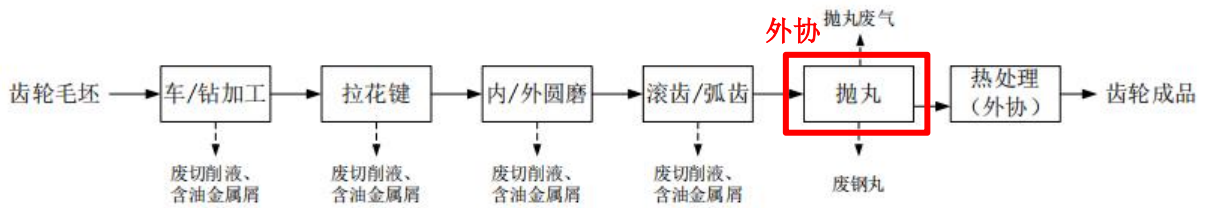
图 2-3 齿轮组生产工艺流程及产污图
